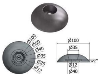
100mm Metec 1kg Disc Anode (MD9Z)
