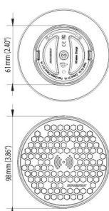
ROKK Wireless Surface - SC-CW-02E
