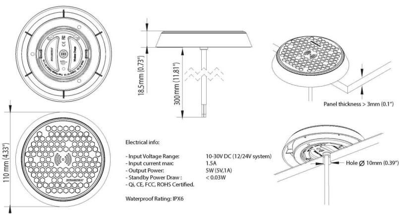
ROKK Wireless Bezel - SC-CW-03E
