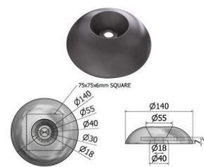
140mm Metec 2.5kg Disc Anode (MD23Z)
