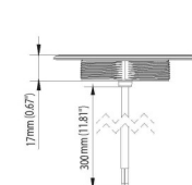
ROKK Wireless Surface - SC-CW-02E
